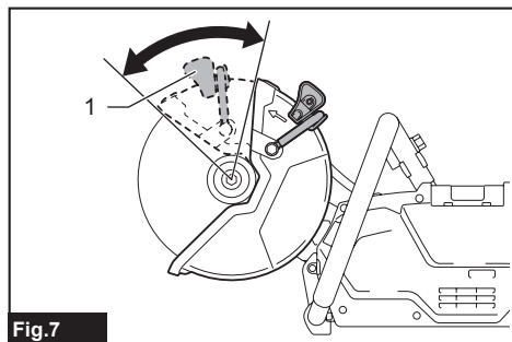
► 1. Empuñadura de la cubierta de la rueda
