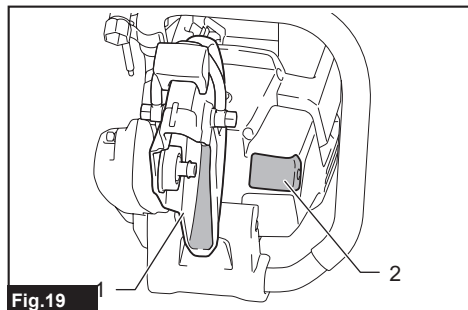
Fig.19 ► 1. Protector de la rueda 2. Lente de la lámpara
