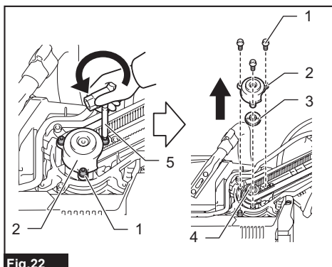
Fig.22 ► 1. Perno de cabeza hexagonal 2. Cubierta 3. Placa 4. Polea (impulsora) 5. Llave de bujías (punta del mango con forma de llave hexagonal)
