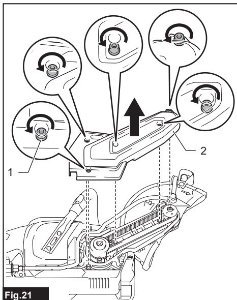
Fig.21 ► 1. Perno de cabeza hexagonal 2. Cubierta
